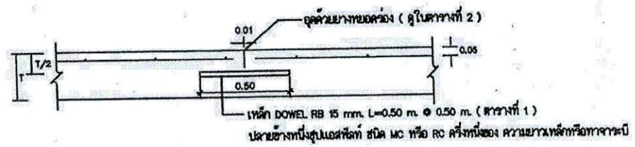
CONTRACTION JOINT (ทุกระยะไม่เกิน 5 ม.)
