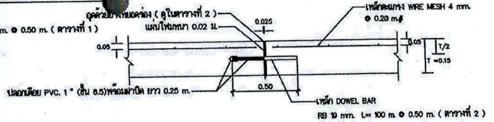
EXPANSION JOINT (ทุกระยะไม่เกิน 50 ม.)
