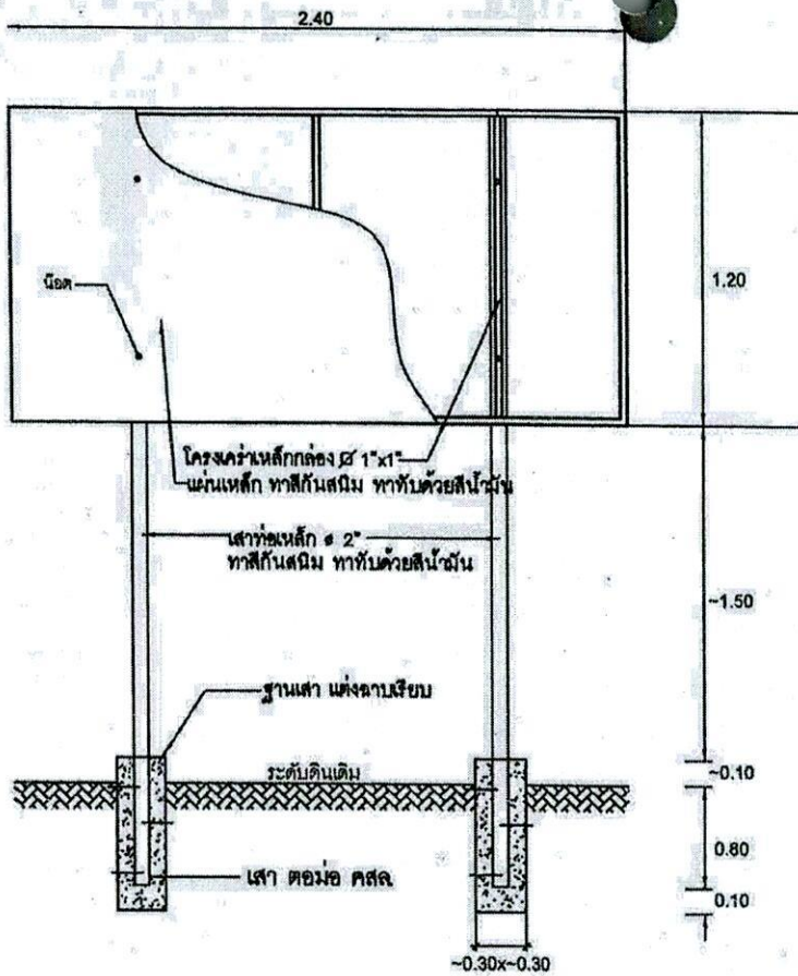
แบบขยายป้ายโครงการ ( ป้ายถาวร )
