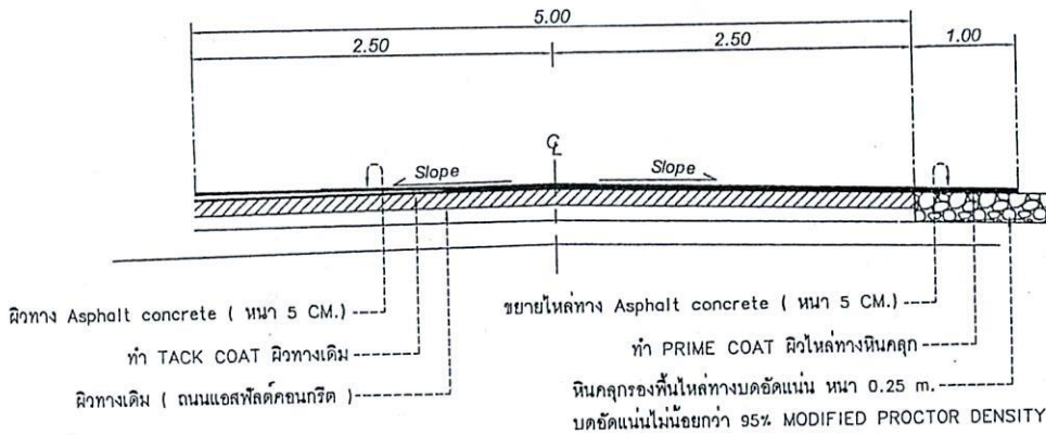
รูปตัดโครงสร้างทาง 1
