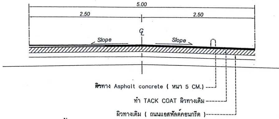
รูปตัดโครงสร้างทาง 1
